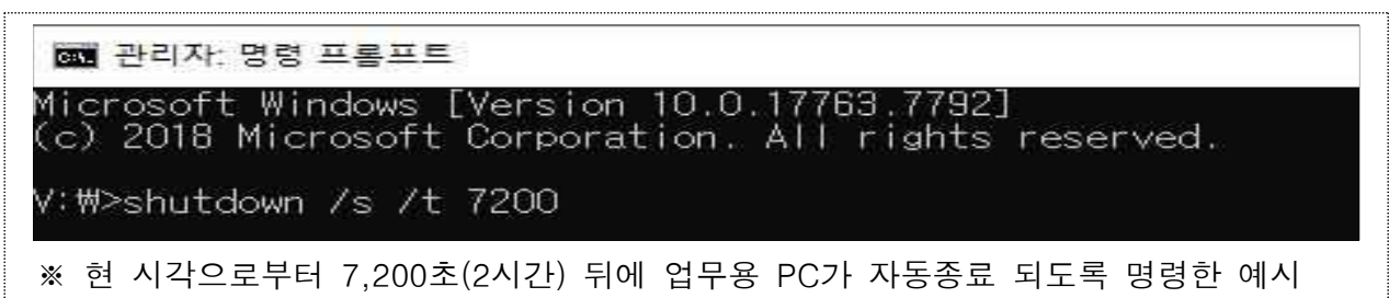
[그림 1] 업무용 PC 자동종료 프로그램 shutdown 구동 예시(화면)
